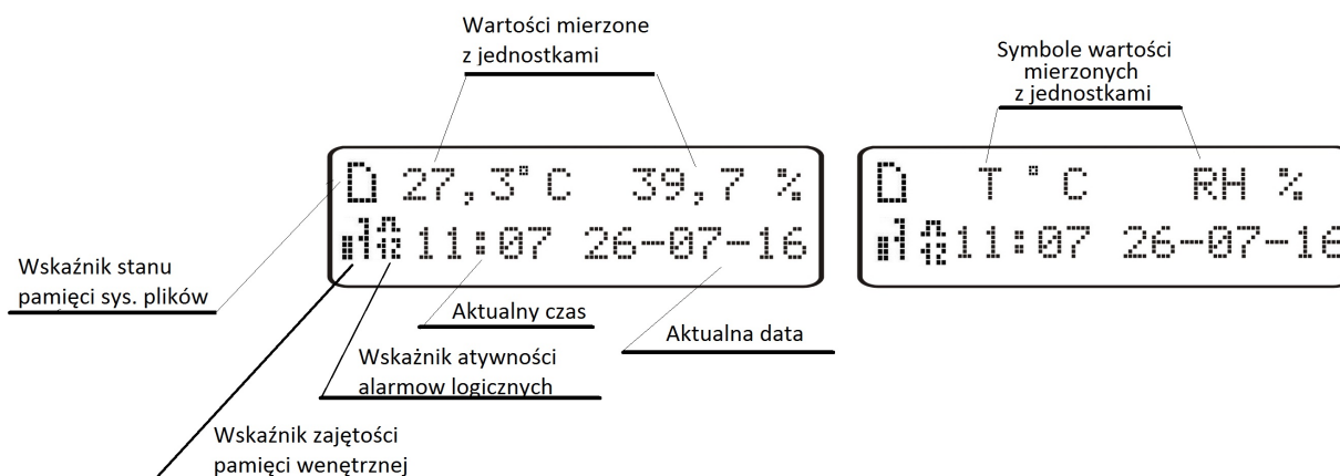
Rys.5. Opis pola odczytowego rejestratora HT20IoT
