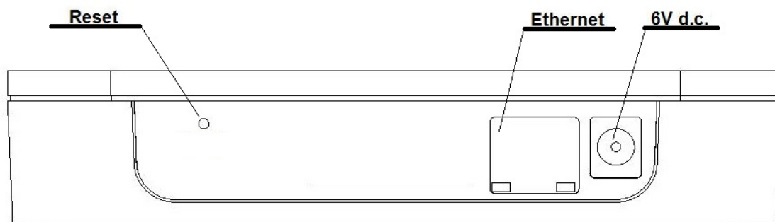
Rys.3. Widok części górnej rejestratora HT20IoT
