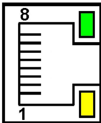
Rys.6. Widok i numeracja pinów gniazda RJ45 rejestratora
